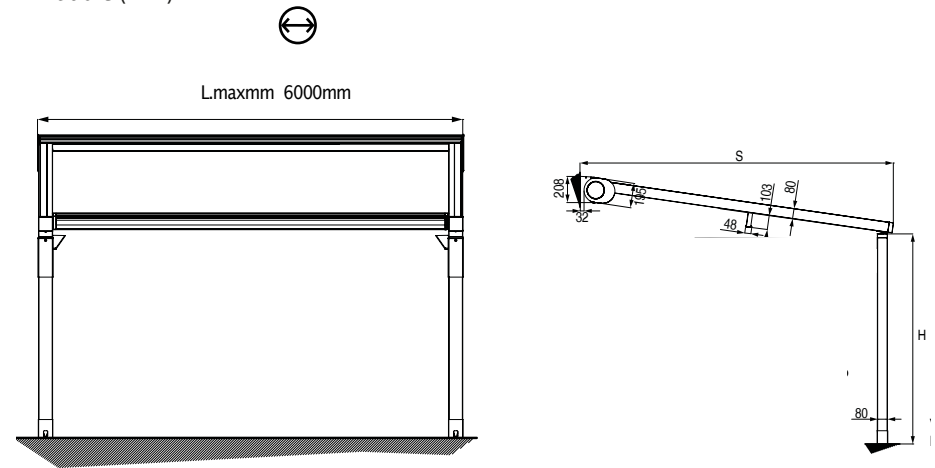
1 Module (mm)
