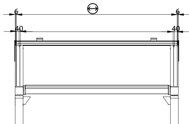
Guides inter axis width (mm)
